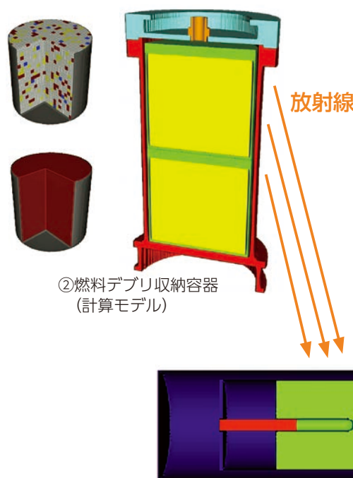
③放射線検出器(計算モデル)
