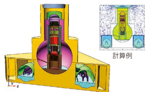
①原子炉格納容器(計算モデル)
